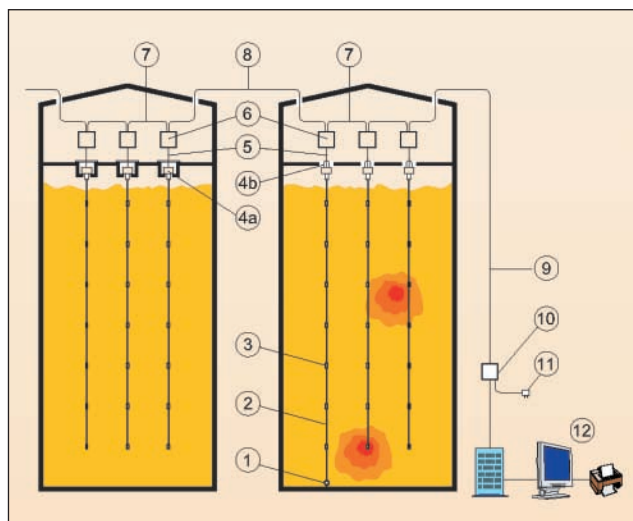
Prinsipp for fjernovervåking i siloer
