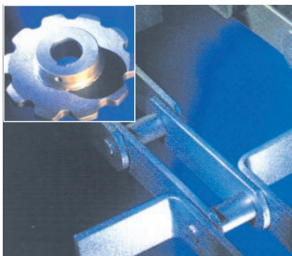
Redlerkjeder og kjedehjul.
